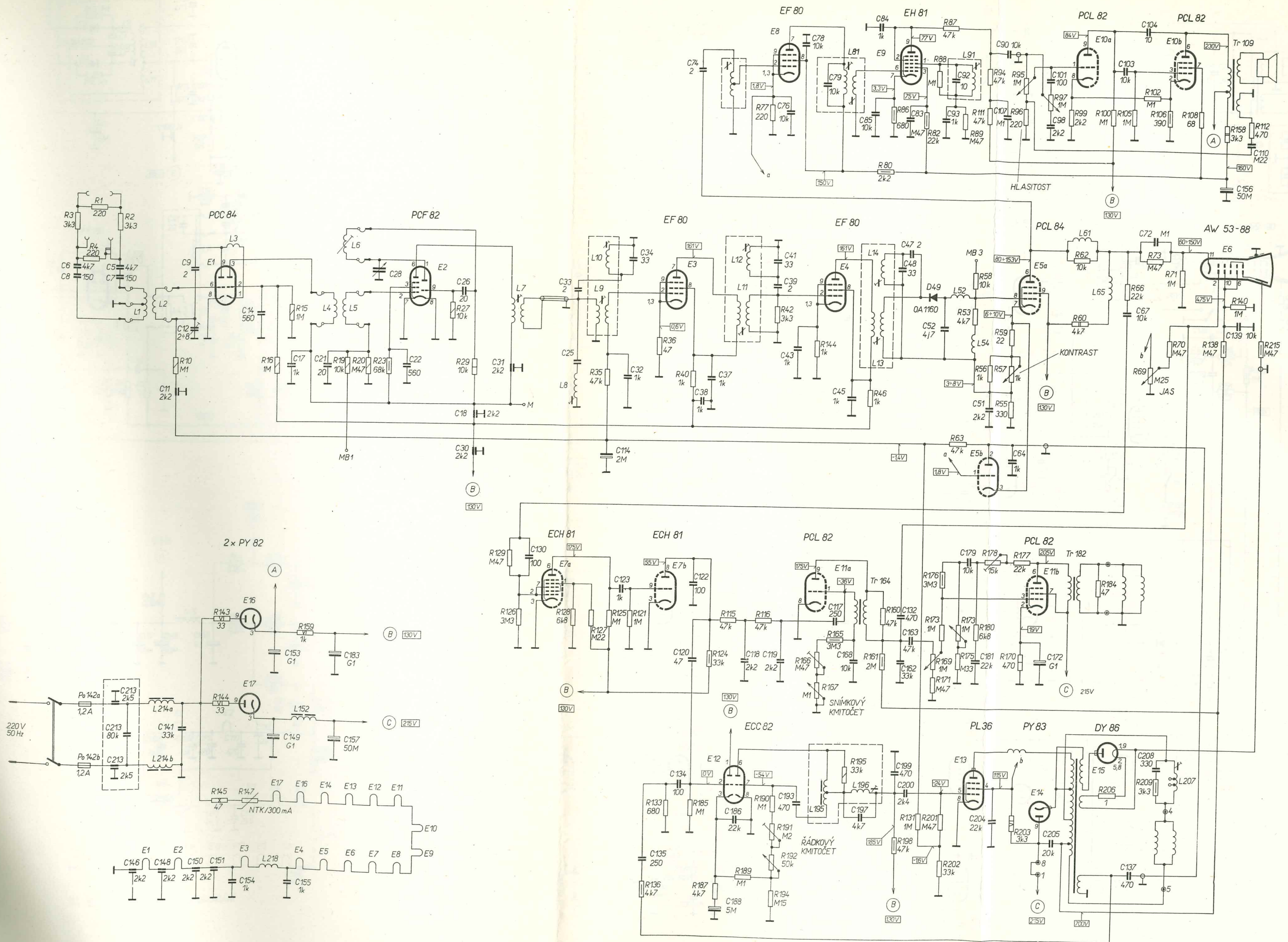
Príloha 9 — Schéma zapojení televízneho prijímače ORION AT 505
