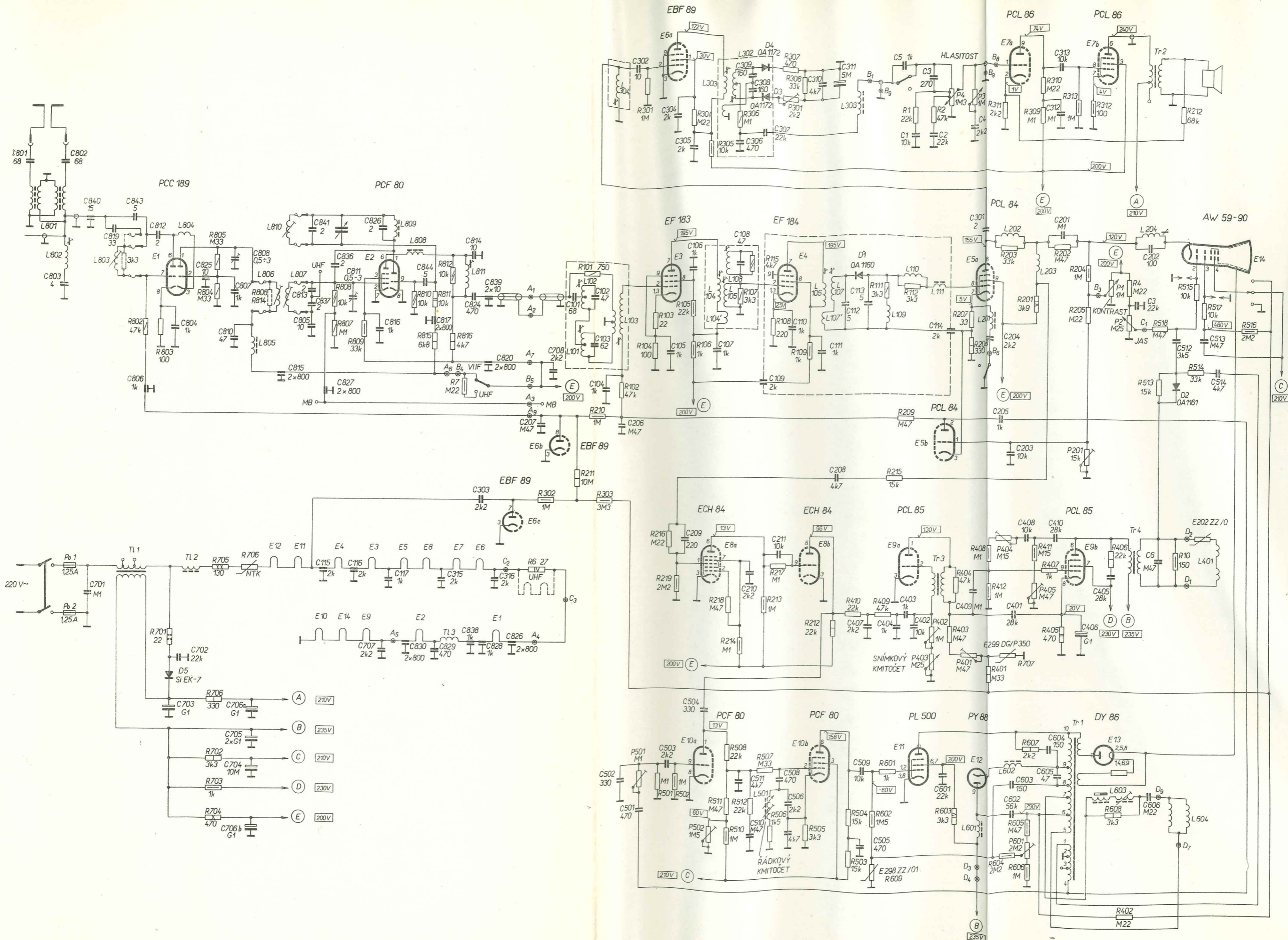
Příloha 14 — Schéma zapojení přijímače AT 550-DELTA
