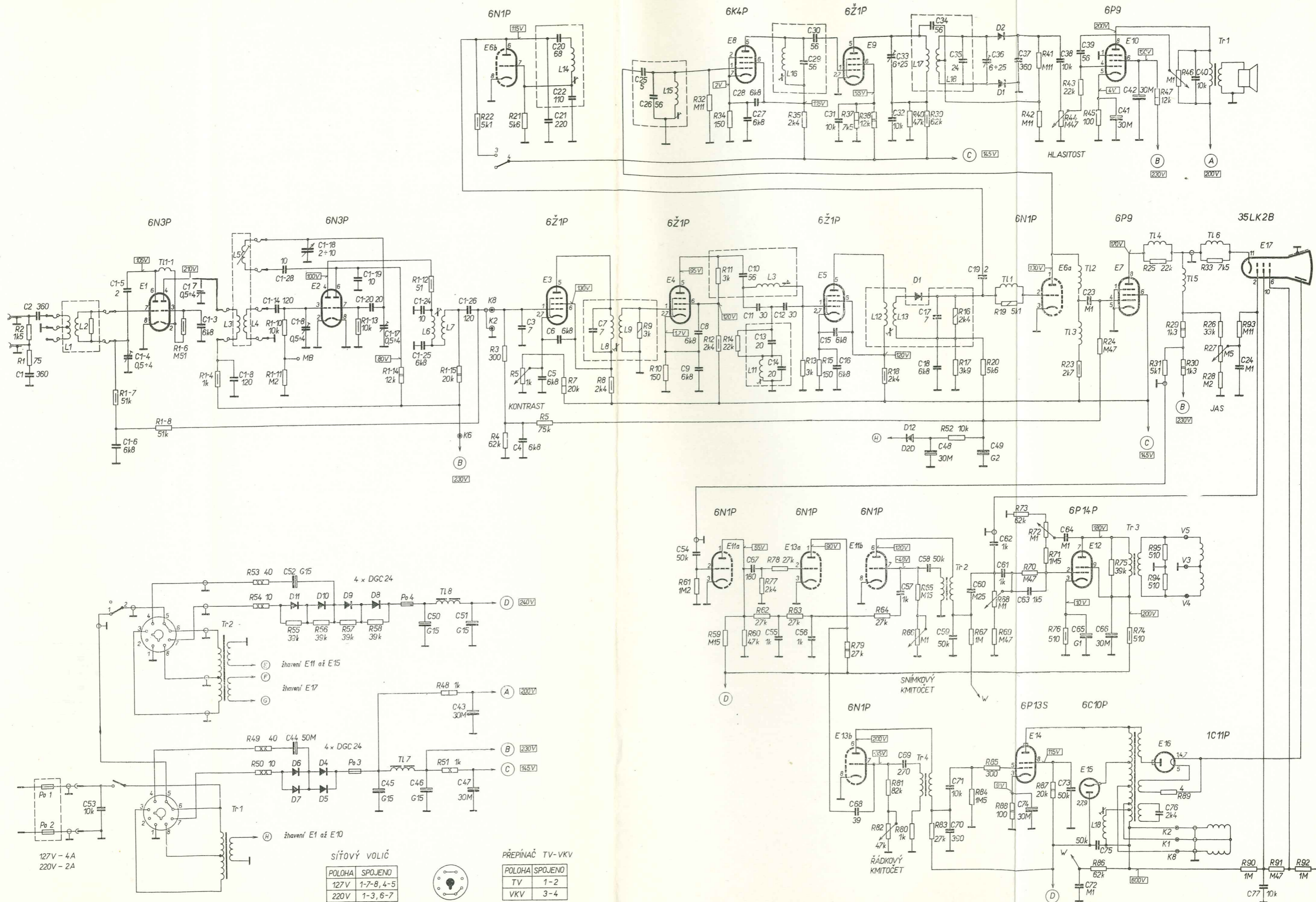
Príloha 16 — Schéma zapojení televizního přijímače REKORD
