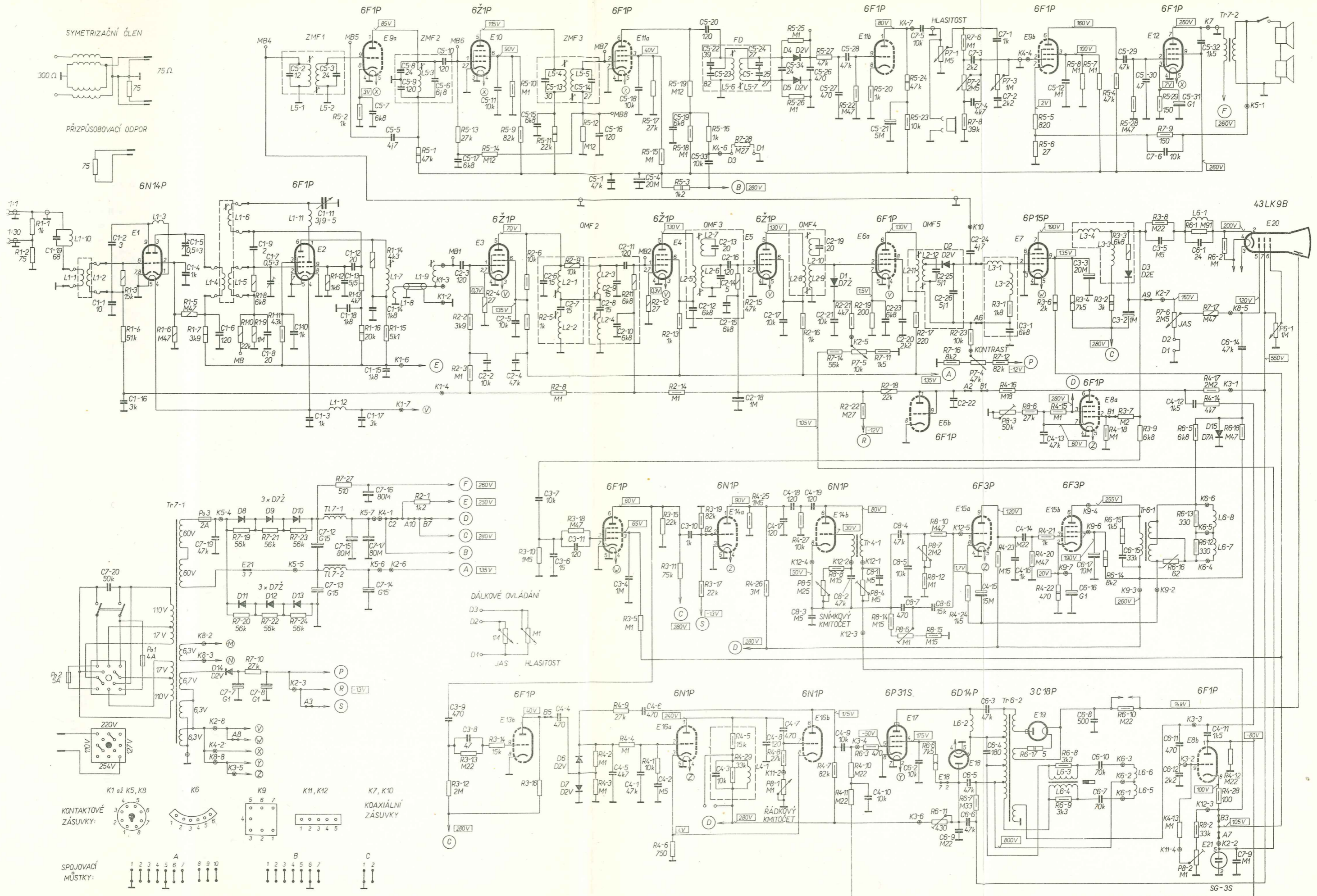
Príloha 23 — Schéma zapojení televizních přijímačů VOLNA ZK 36 a SIGNAL
