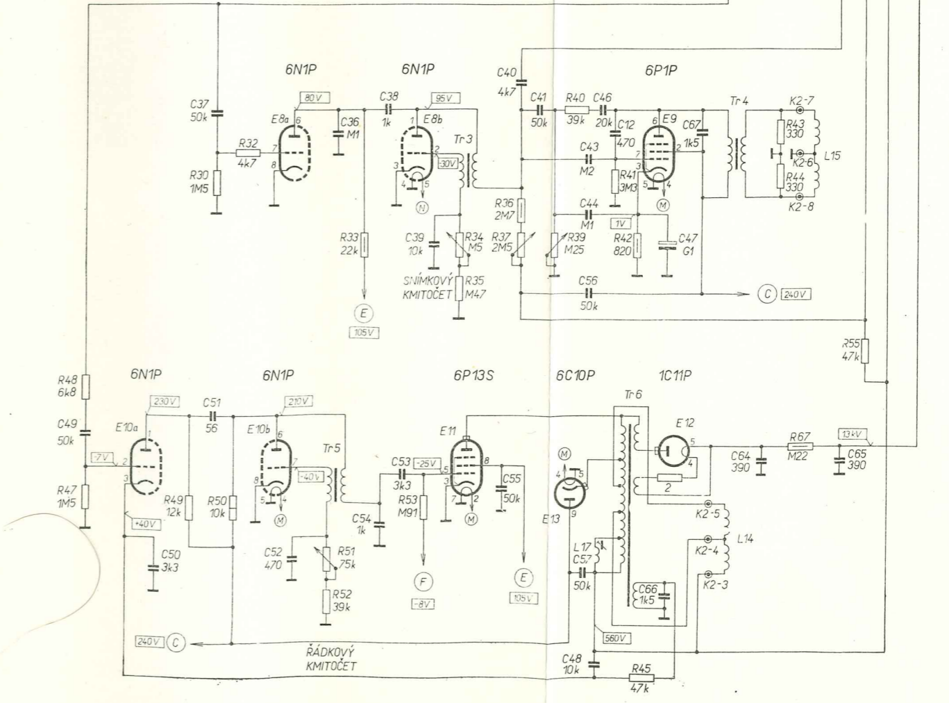
Príloha 22 — Schéma zapojení televizního přijímače ZNAMJA 58
