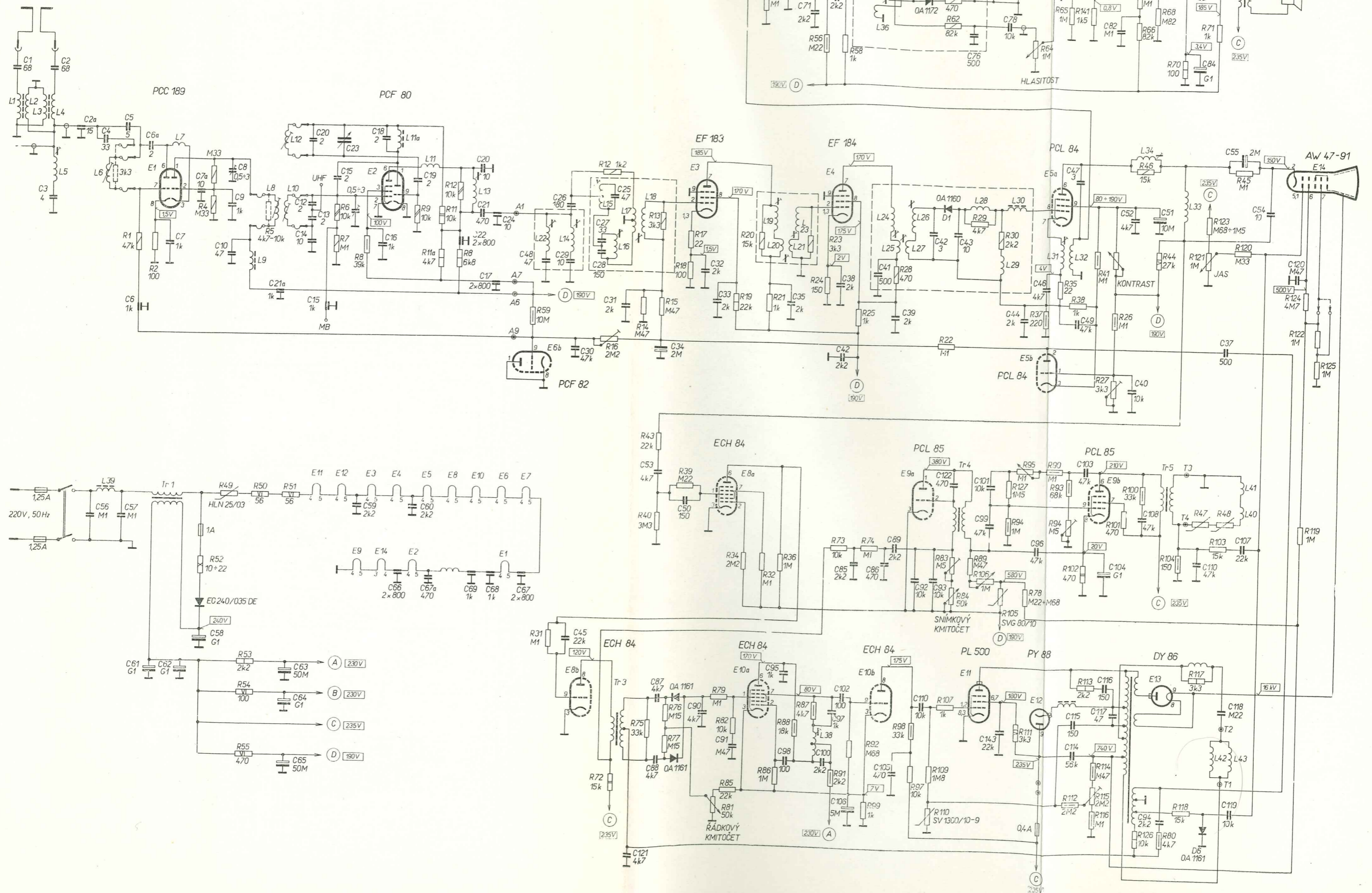
Příloha 13 — Schéma televizního přijímače FAVORIT
