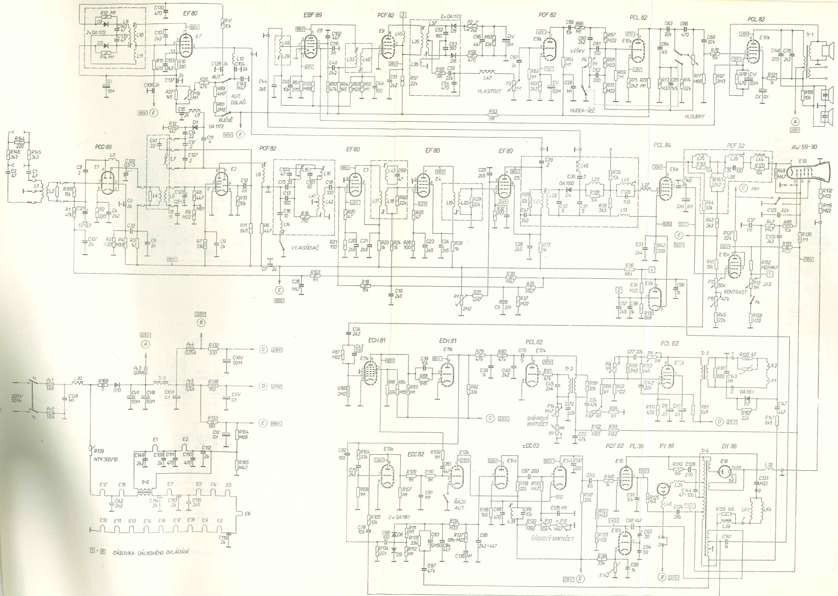
Příloha 10 – Schéma zapojení televizního přijímače ORION AT 611
