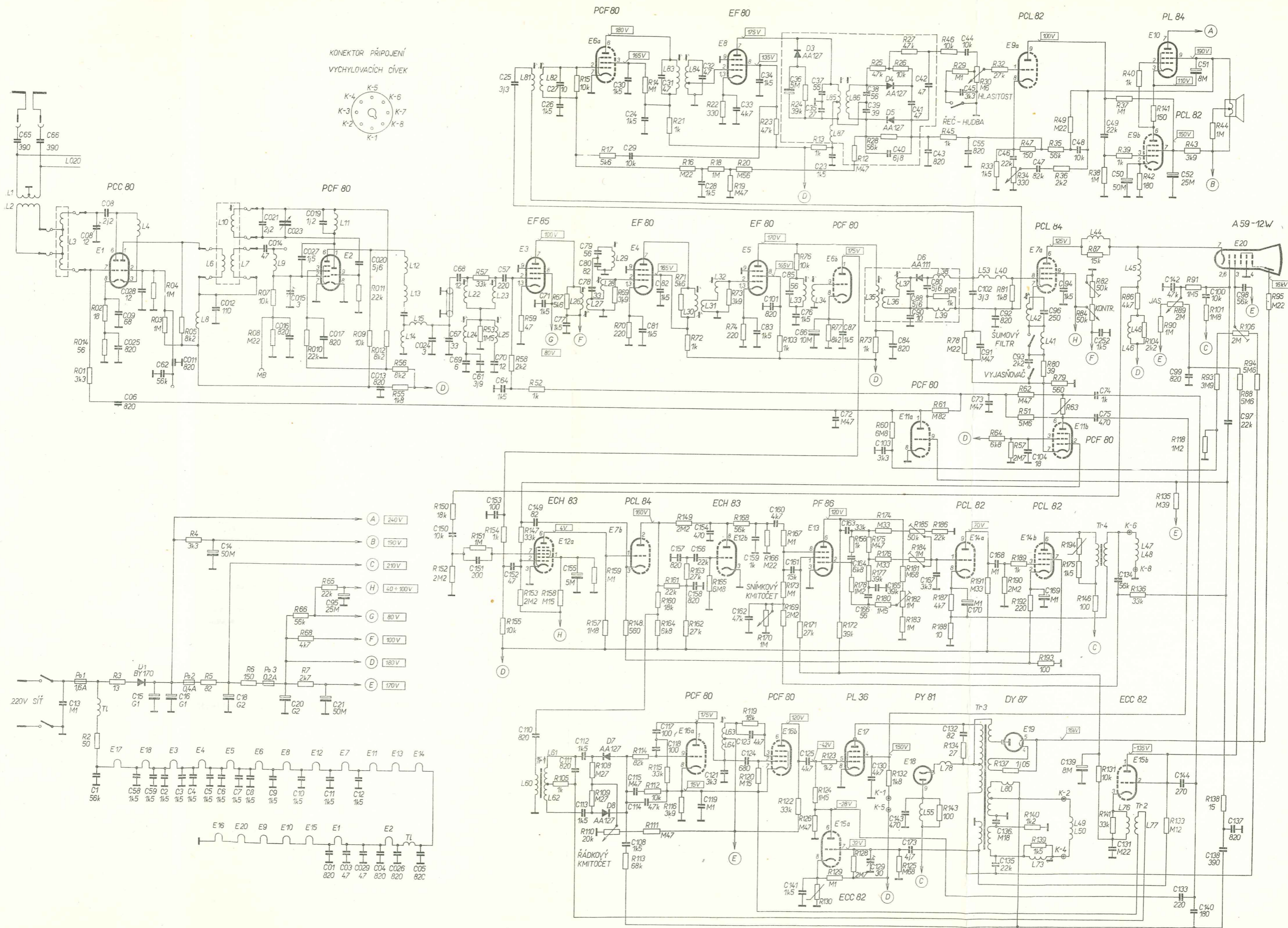
Příloha 24 — Schéma zapojení přijímače NIŠAVA a SÁVA (Elektronka E1 je správně PCC 88)
