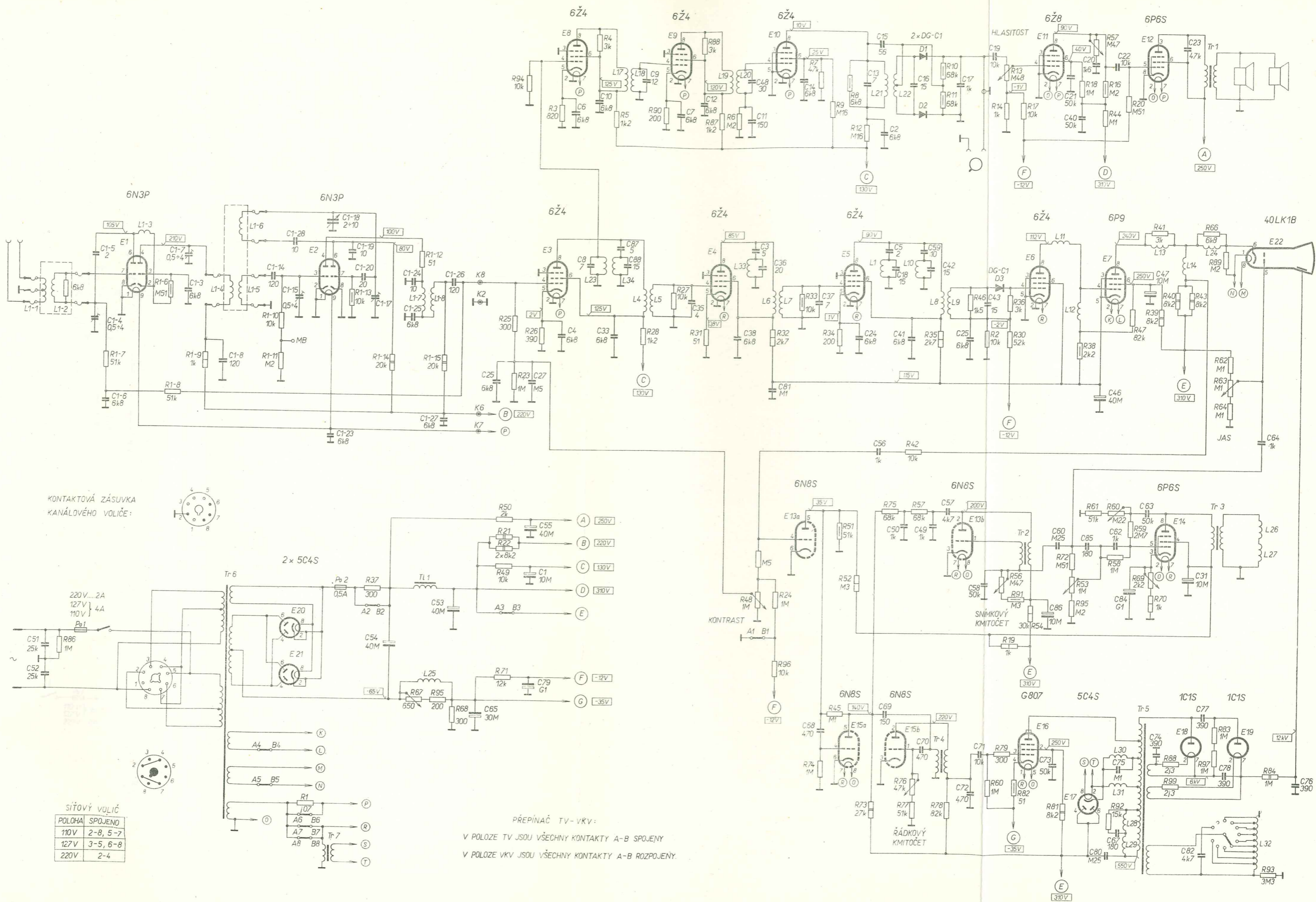
Příloha 19 – Schéma zapojení televizního přijímače Temp 2
